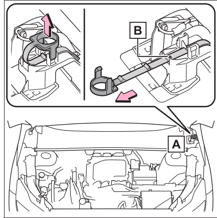
A Notentriegelungshebel
